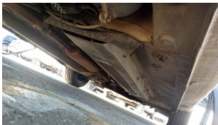
Estrutura Assoalho
